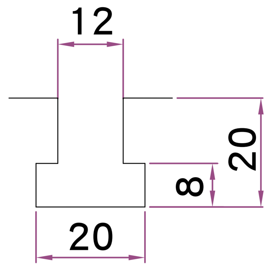
T 型槽尺寸
