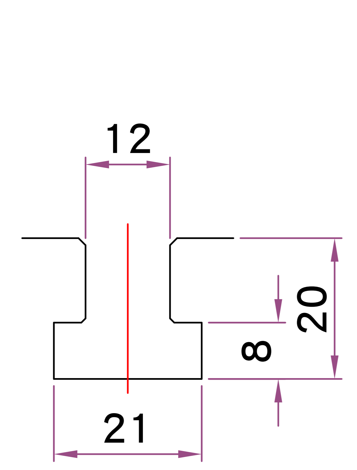
T 型槽尺寸
