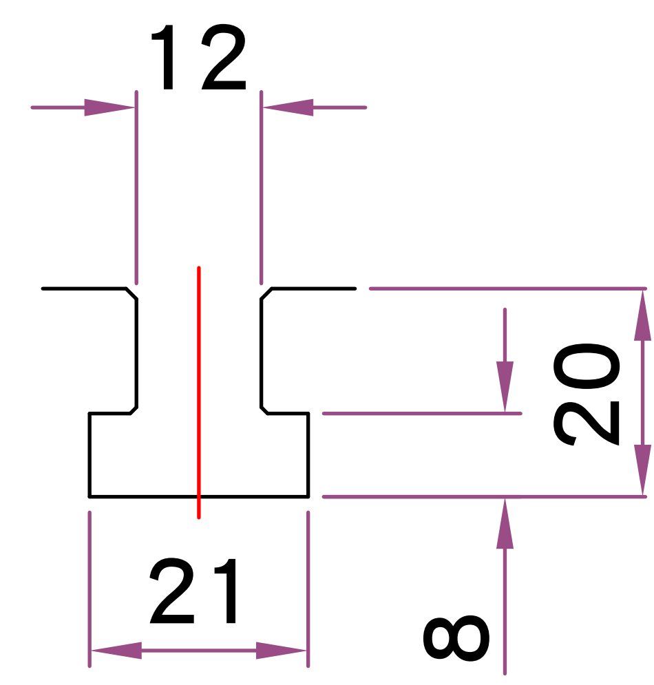
T 型槽尺寸
