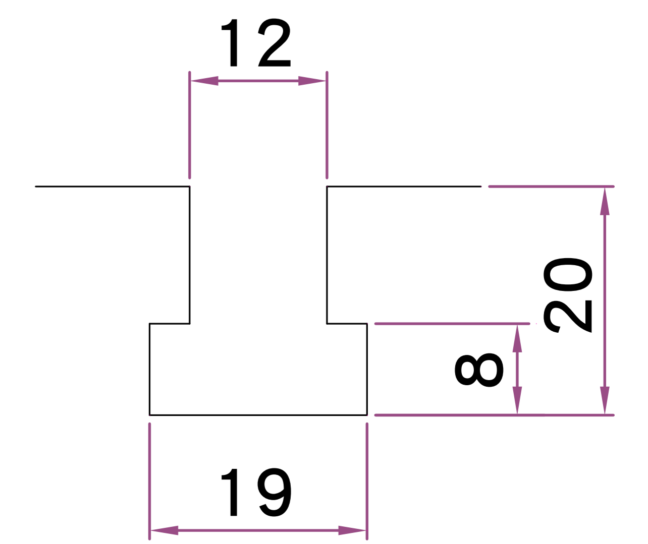
T 型槽尺寸
