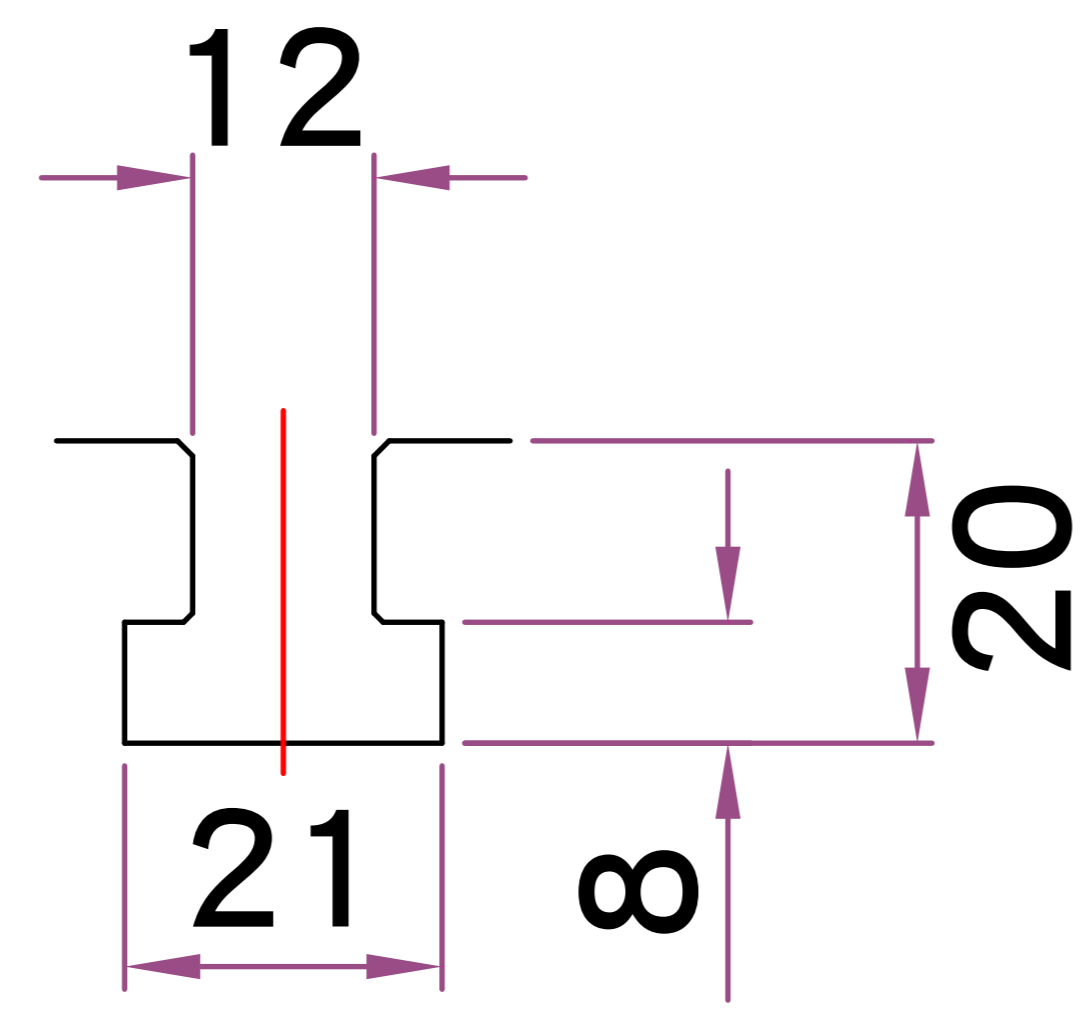
T 型槽尺寸
