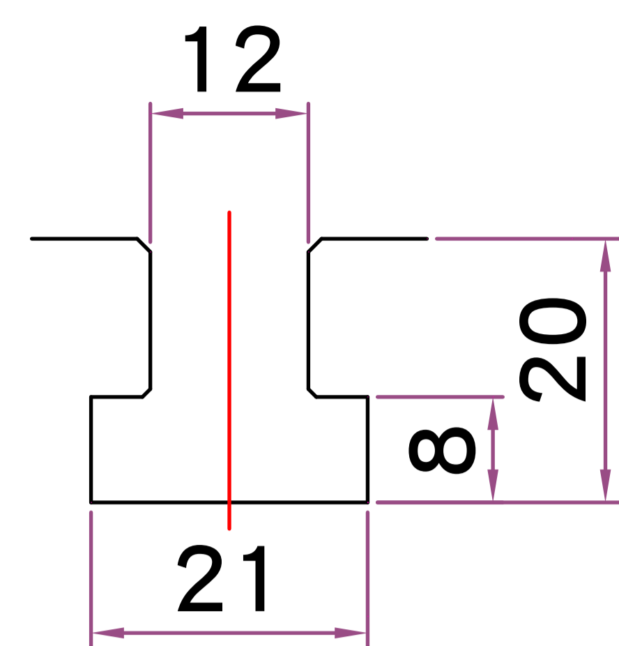
T 型槽尺寸
