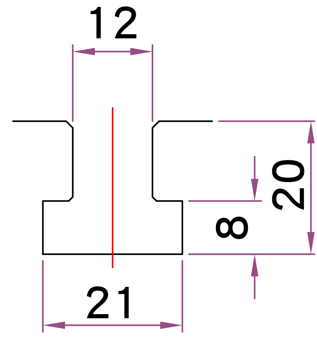
T 型槽尺寸
