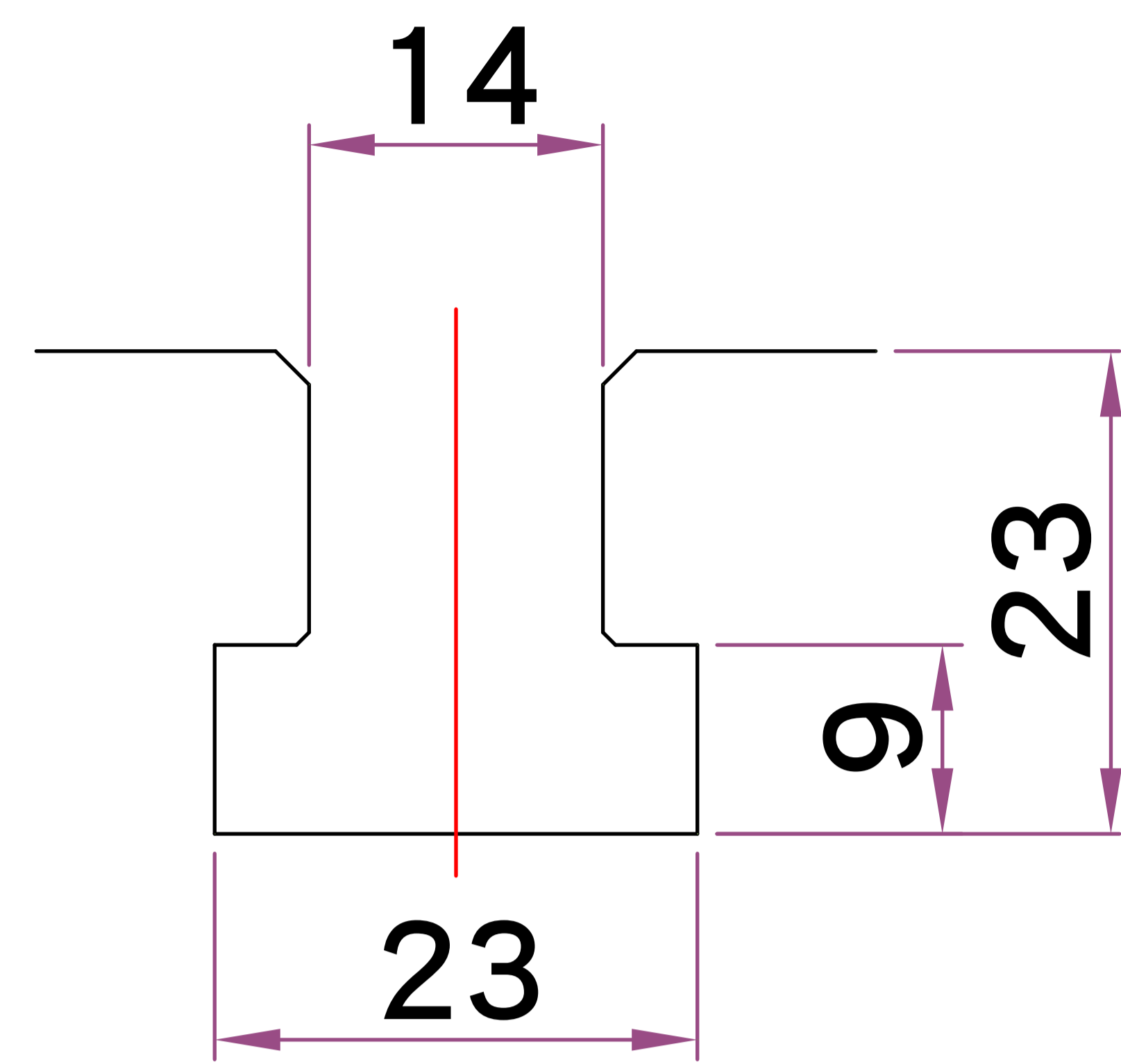
T 型槽尺寸
